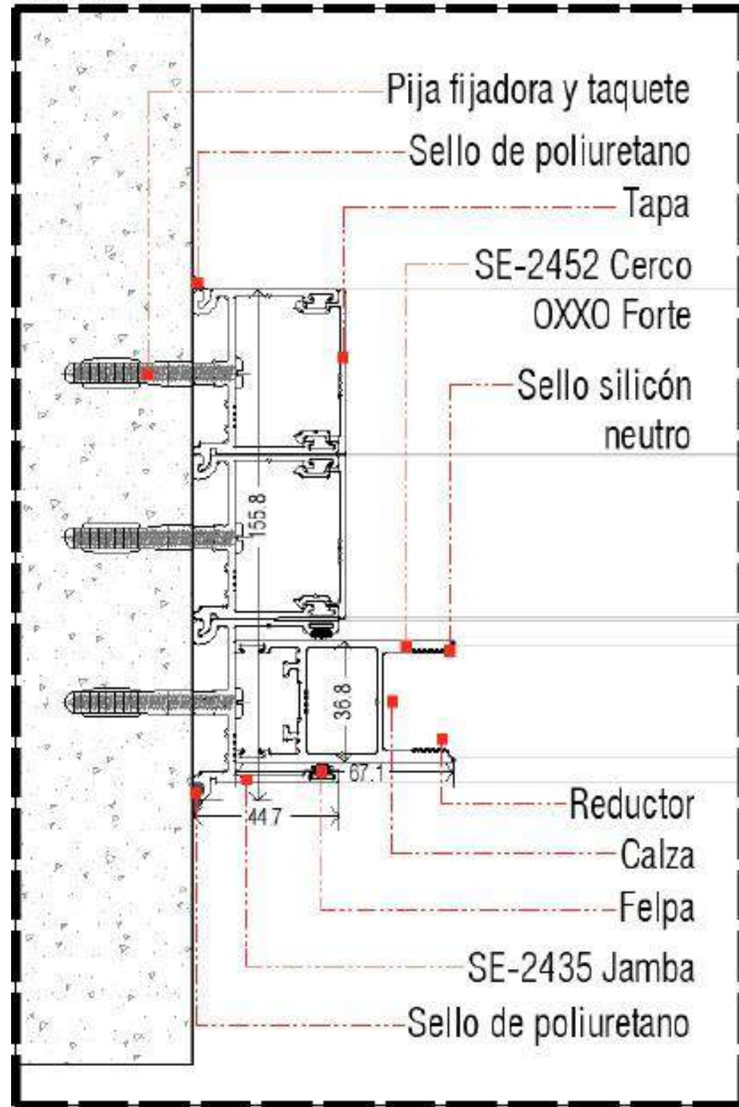
Corte A
